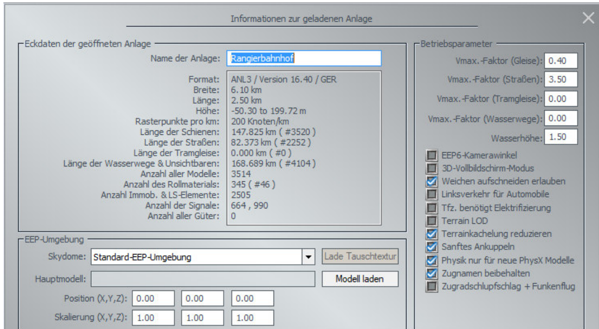
Fig.1 : Informations système
